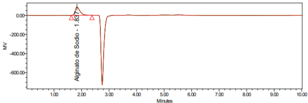
Figura 2. Cromatograma característico de la solución estándar.
